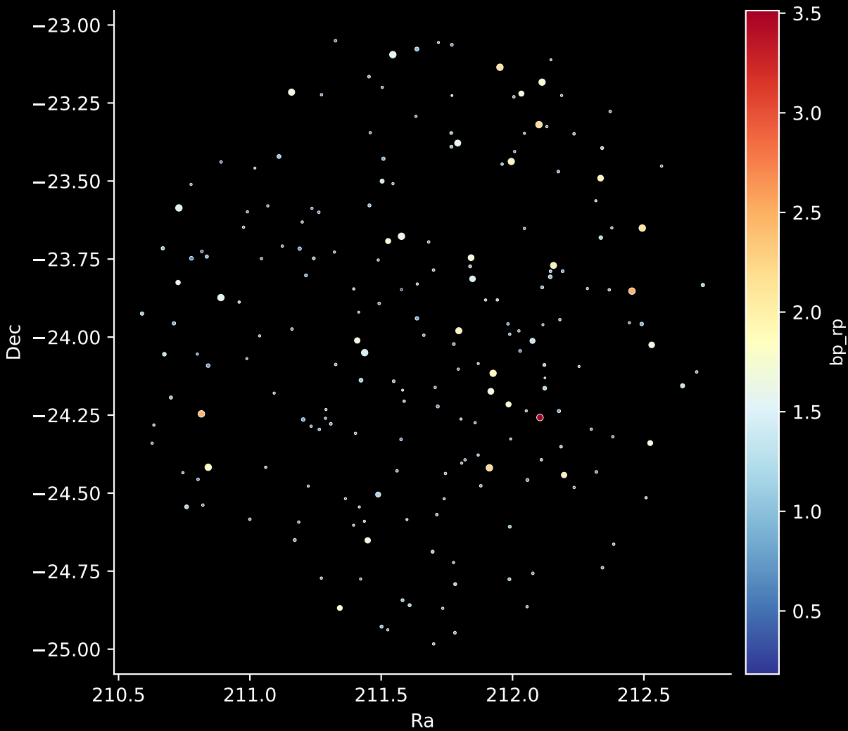
GALAH DR4 Field: [8439] Stars: 206
