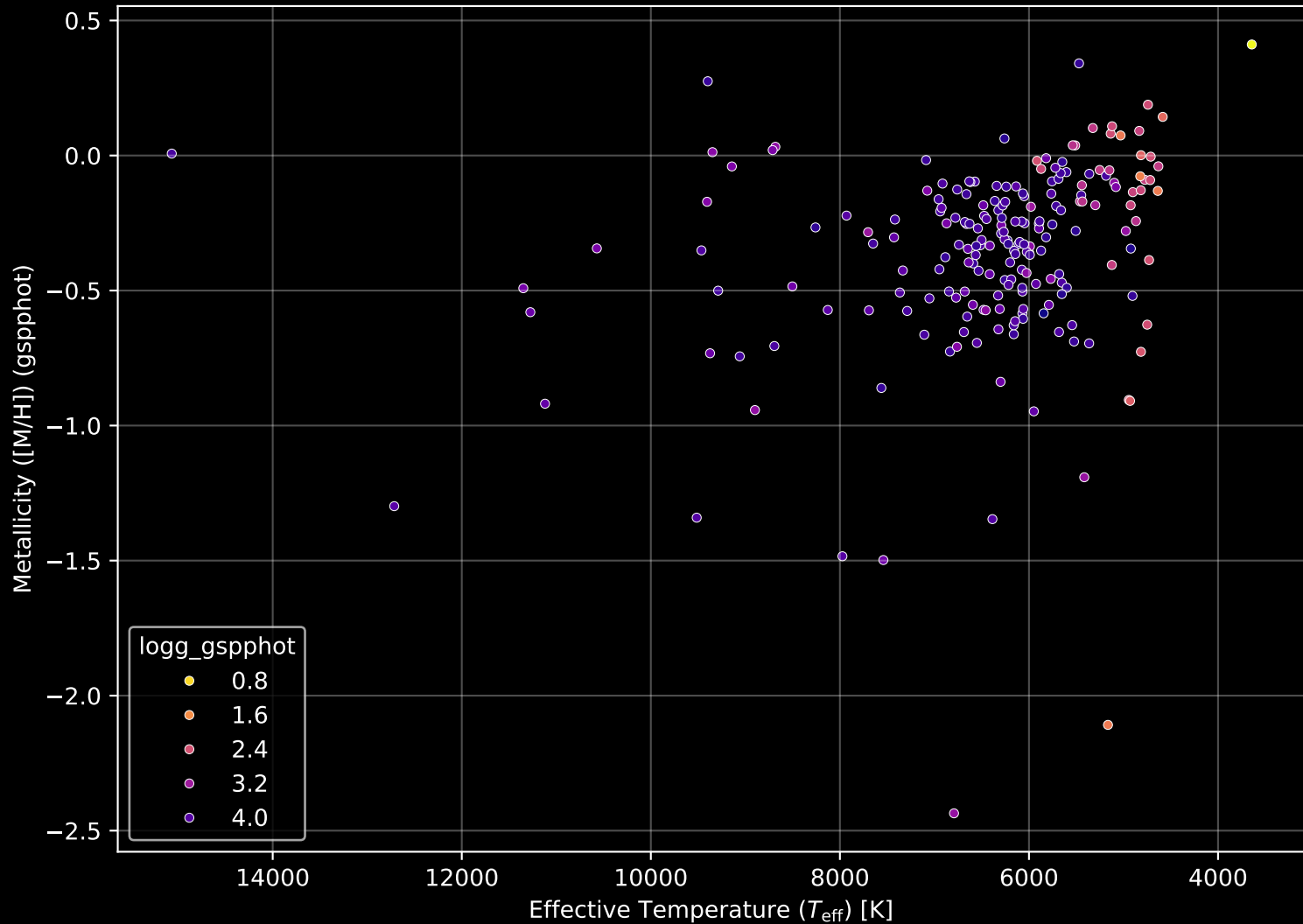
GALAH DR4 Field: [8439] Stellar Population Parameters (n= 206)
