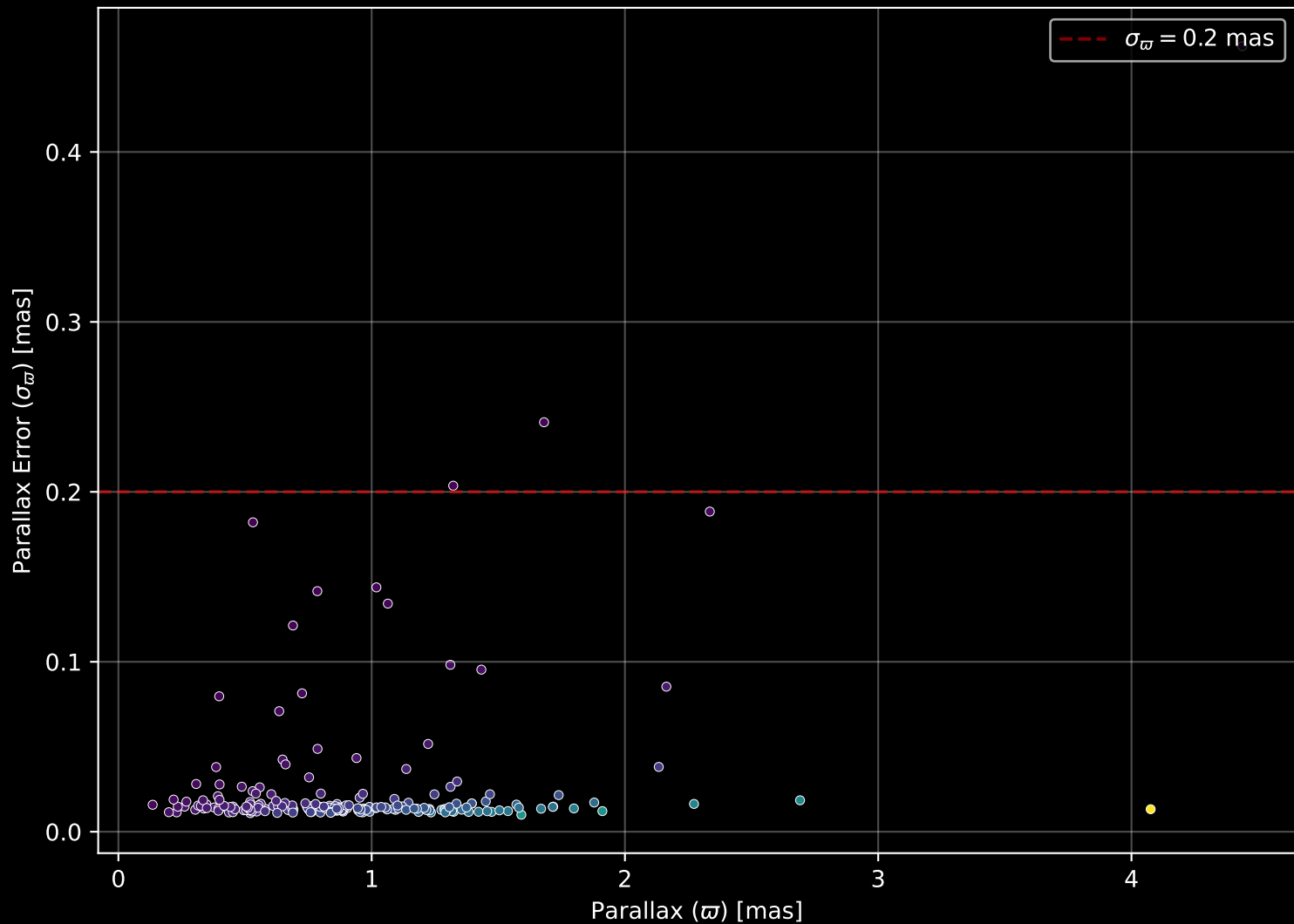
GALAH DR4 Field: [8439] Parallax Quality (n= 206)
