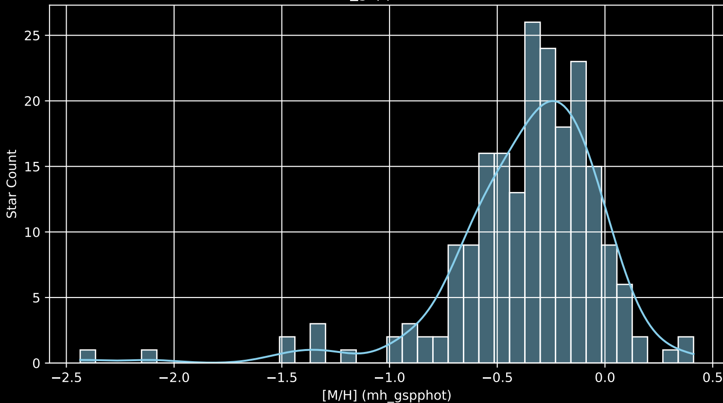
GALAH DR4 Field: [8439] [M/H] (mh_gspphot) (n= 206)
